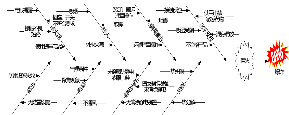
图 3-1 烟花爆竹储存库发生火灾、烟花爆竹爆炸事故的因果分析图
